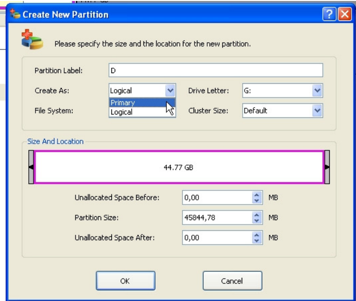
02)_kreiranje nove particije
