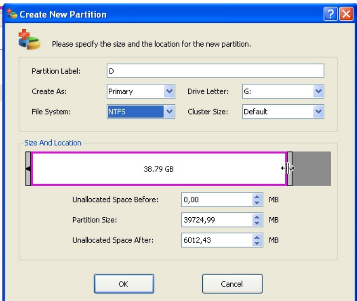
04)_kreiranje nove particije
